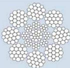
8x19W - IWRC
