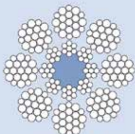
8 x 19 W - IWRC
