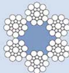
6 x 19 S - FC
